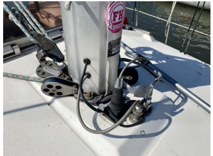
Mast / Mastfuß Ansicht 2
